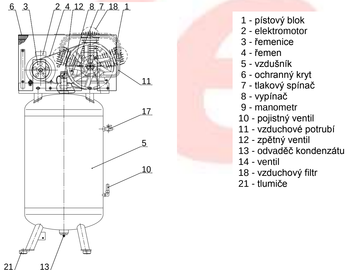
Obr. 6 - Celkový pohled na kompresor F-270.LB75V
