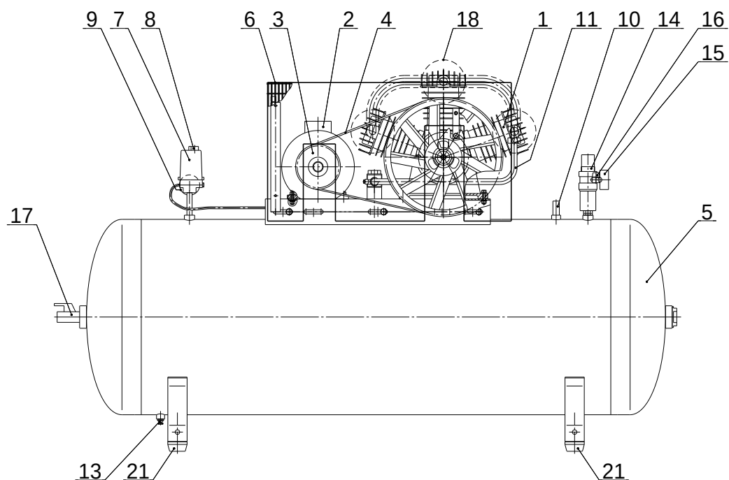
Obr. 7 - Celkový pohled na kompresor F-500.LB75
