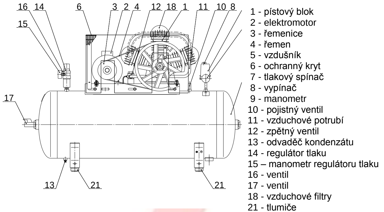
Obr. 5 - Celkový pohled na kompresor F-270.LB75
