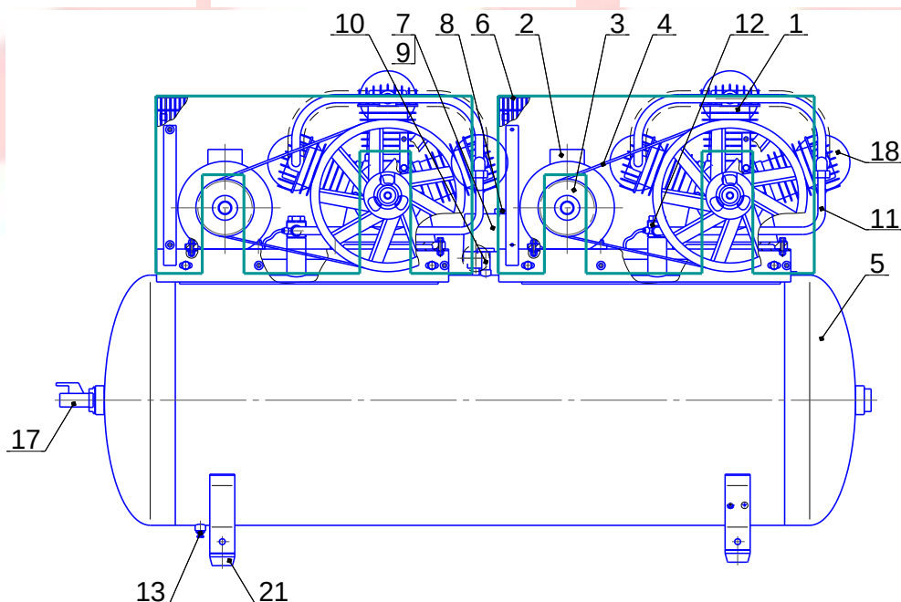
Obr. 8 - Celkový pohled na kompresor F-500.LB75TB
