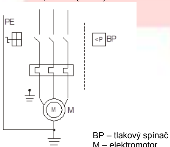
Obrázek A.2 – Schéma elektrických obvodů kompresoru F-500.LB75TB
