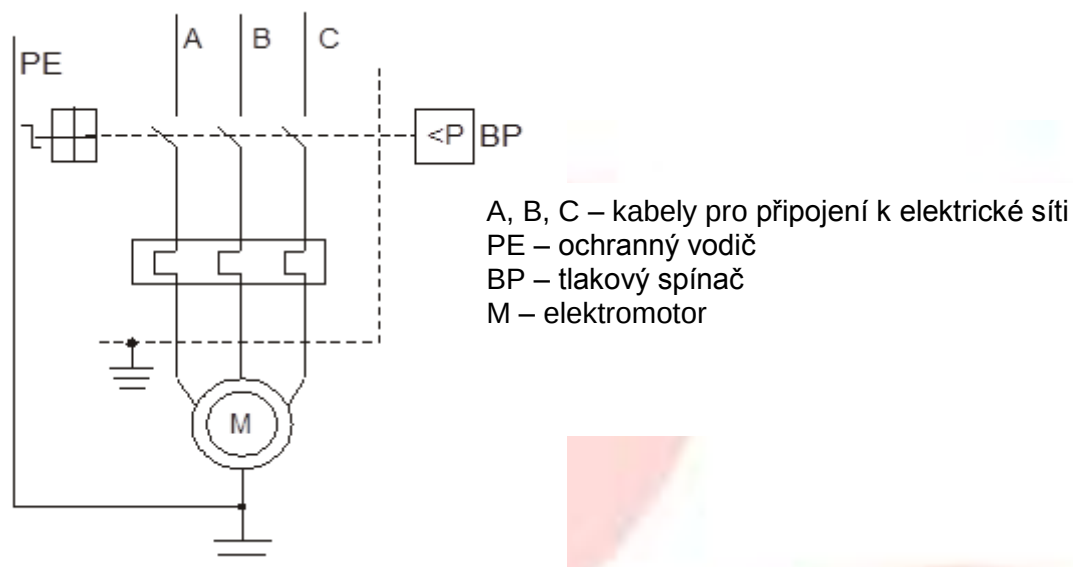
Obrázek A.1 – Schéma elektrických obvodů kompresorů C-100.LB75, F-570.LB75, F-270.LB75V, F-500.LB75
