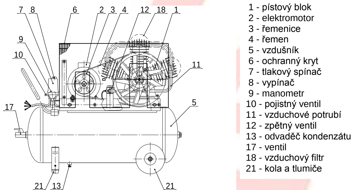
Obr. 4 - Celkový pohled na kompresor C-100.LB75
